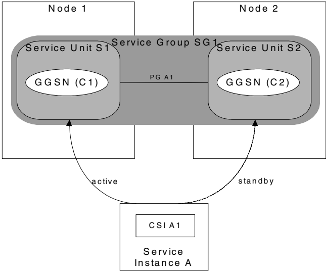
Fig. 3. SA Forum system model entities
